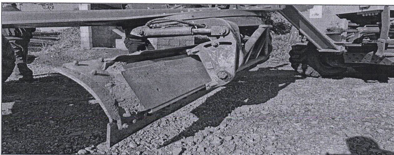
IMAGEM GERAL DA LÂMINA DA MOTONIVELADORA, RECOMPOSIÇÃO DO EMBUCHAMENTO DEVE SER REALIZADO
