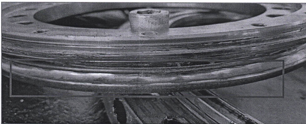
IMAGEM DETALHADA DE ROLAMENTO DO TÂNDEM, SINAIS DE DESGASTE, MARCAÇÃO DAS ESFERAS VISÍVEIS
