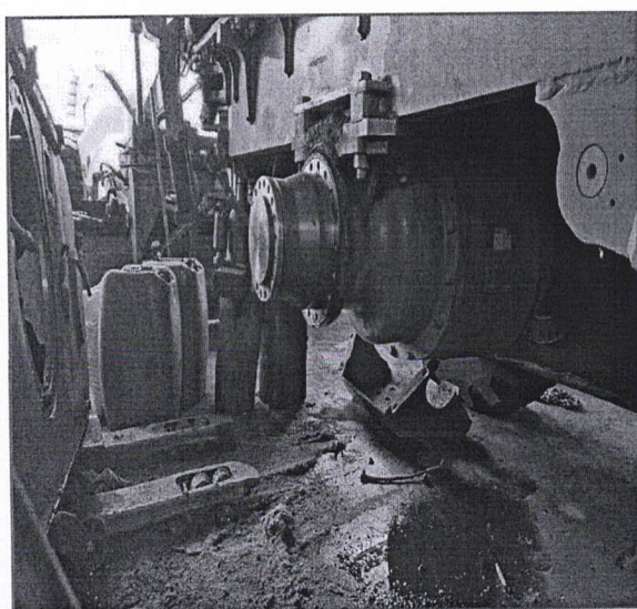
IMAGENS DA MOTONIVELADORA JÁ DESMONTADA PARA VERIFICAÇÃO DOS TÂNDENS
