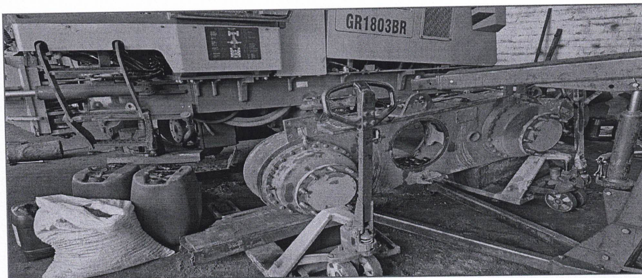
IMAGEM DA MOTONIVELADORA JÁ DESMONTADA PARA VERIFICAÇÃO DOS TÂNDENS
