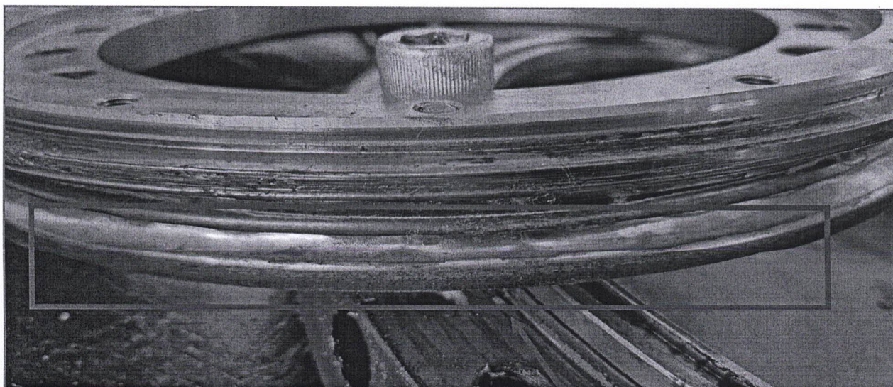
IMAGEM DETALHADA DE ROLAMENTO DO TÂNDEM, SINAIS DE DESGASTE, MARCAÇÃO DAS ESFERAS VISÍVEIS
