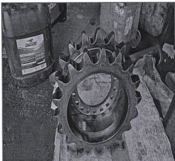
IMAGEM DE ENGRENAGENS E ROLAMENTOS DOS TÂNDENS JÁ DESMONTADOS PARA VERIFICAÇÃO
